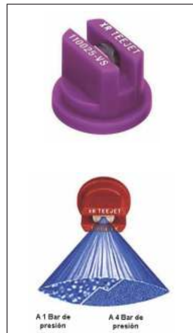
Figura 5. Pastillas de abanico plano de rango extendido.
