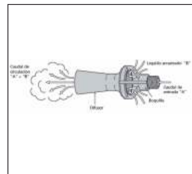
Figura 4: Agitador hidráulico o “eductor”
