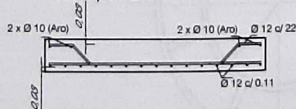
Corte por B-B'
