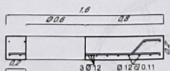
Corte por B-B'
