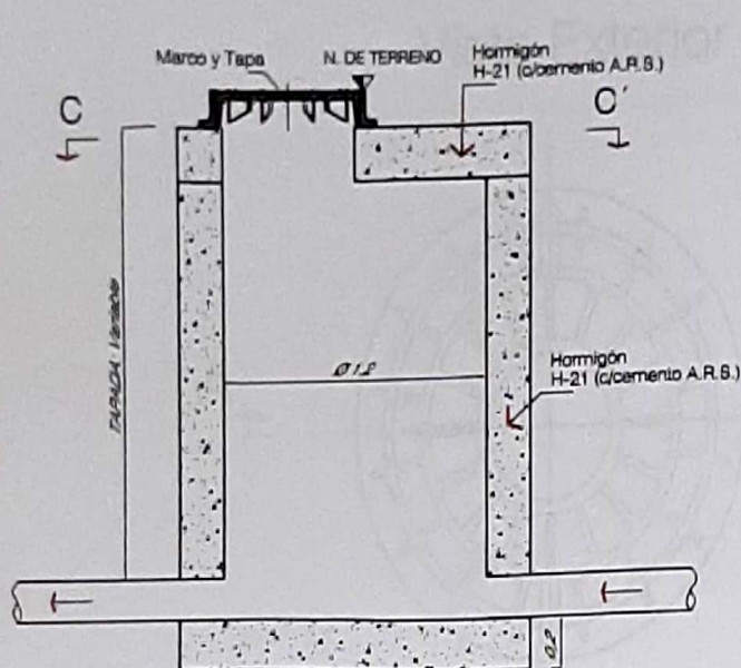
Corte por C-C'
