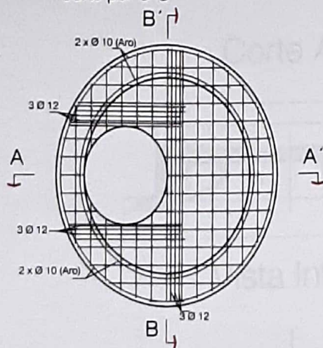
Corte por A-A'
