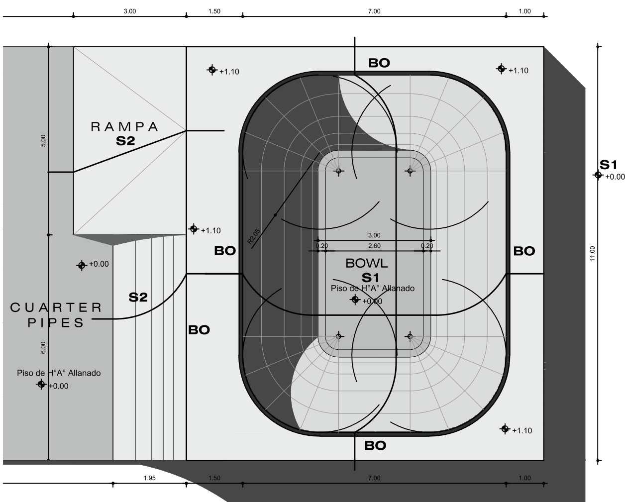
Plano Sector 3 - Esc 1:100
